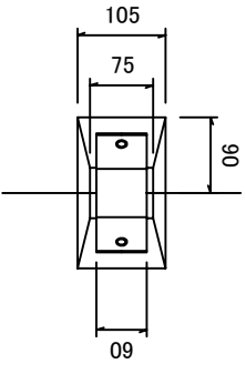
連結部詳細図
