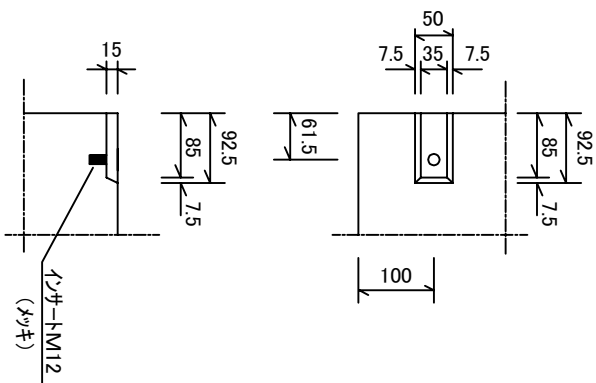
連結部詳細図 S=1/10
