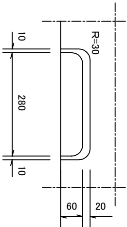
水抜き穴拡大図 S=1/10
