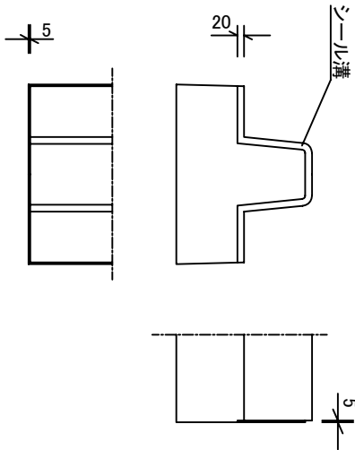
ジョイント部 詳細図 S=1/20
