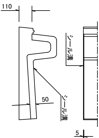
ジョイント部 詳細図 S=1/200
