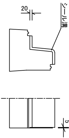
ジョイント部 詳細図 S=1/20
