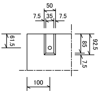
連結部詳細図 S=1/10
