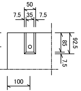
連結部詳細図 S=1/10
